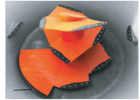
Nuestro Sinfin reforzado está fabricado completamente en chapa 5/8 con más de 16 pliegues que generan mayor robustez.
