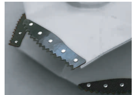
Cuchillas diseñadas por Industrias RENO, de 54cm. diente serrucho cementadas para su autoafilado y mayor duración.
